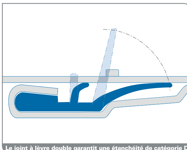
Le joint à lèvres double garantit une étanchéité de catégorie D
